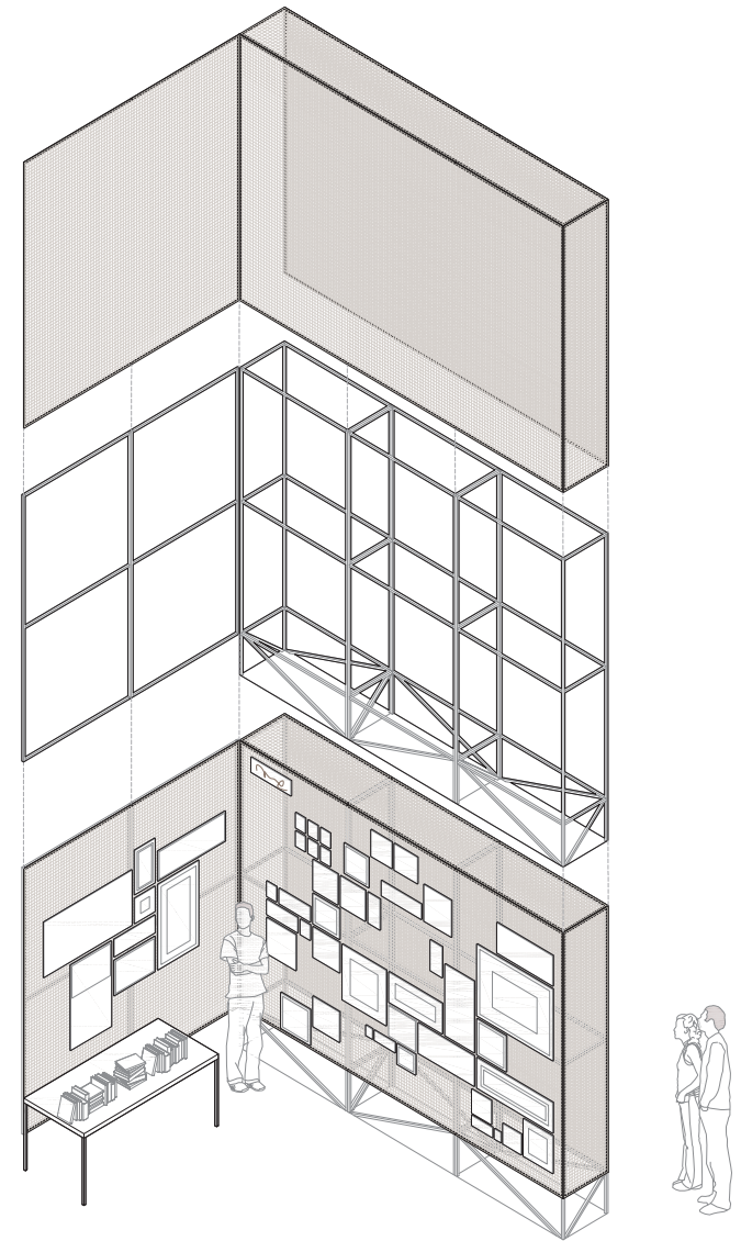
Axonometría de montaje de un Gabinetete tipo
